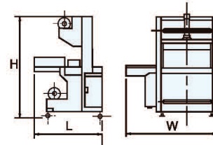
機械尺寸圖 M / C Dim. Illustration
