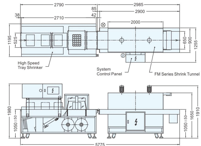
機械外觀尺寸圖 / M/C Dim. Illustration 單位 / mm
